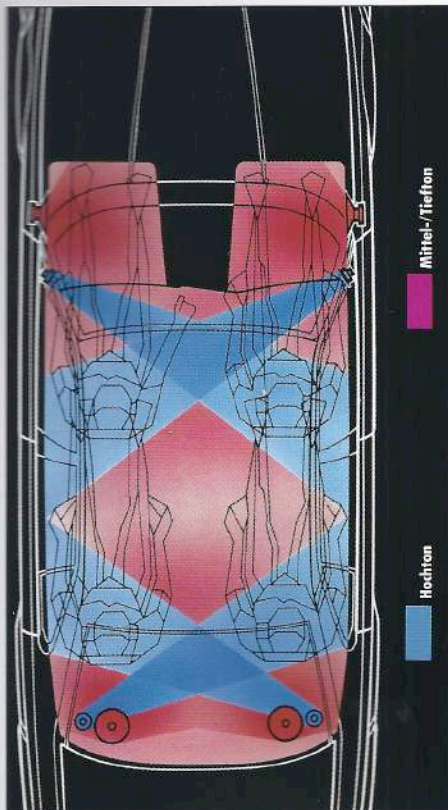
④ BMW Sound-System, 8 Hochleistungs-lautsprecher und Zusatzendstufe mit 4 x 15 Watt Sinus Ausgangsleistung. Perfekte Technik für ein vollendetes Klangerlebnis, speziell auf Ihren BMW 3er abgestimmt.
