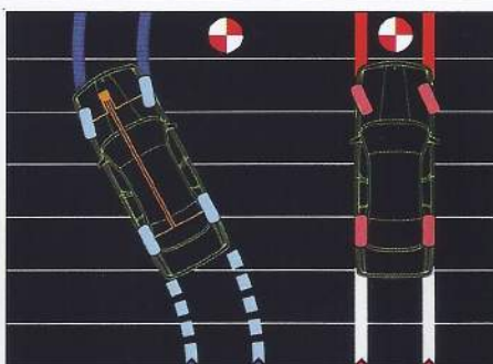
⑤③ Anti-Blockier-System (ABS). Das BMW ABS bietet optimale Sicherheit beim Bremsen auf kritischem Untergrund.
